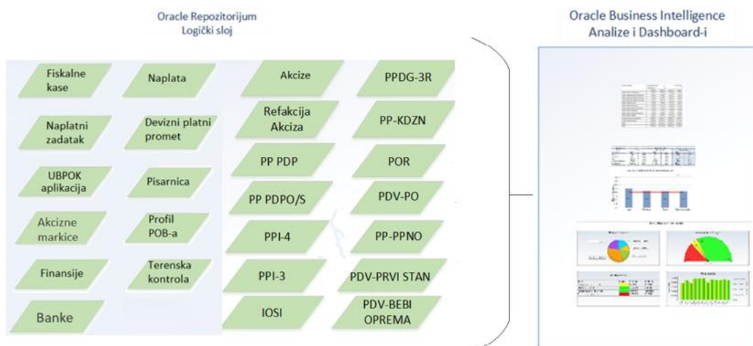
Илустрација 2: Пословна архитектура DWH
