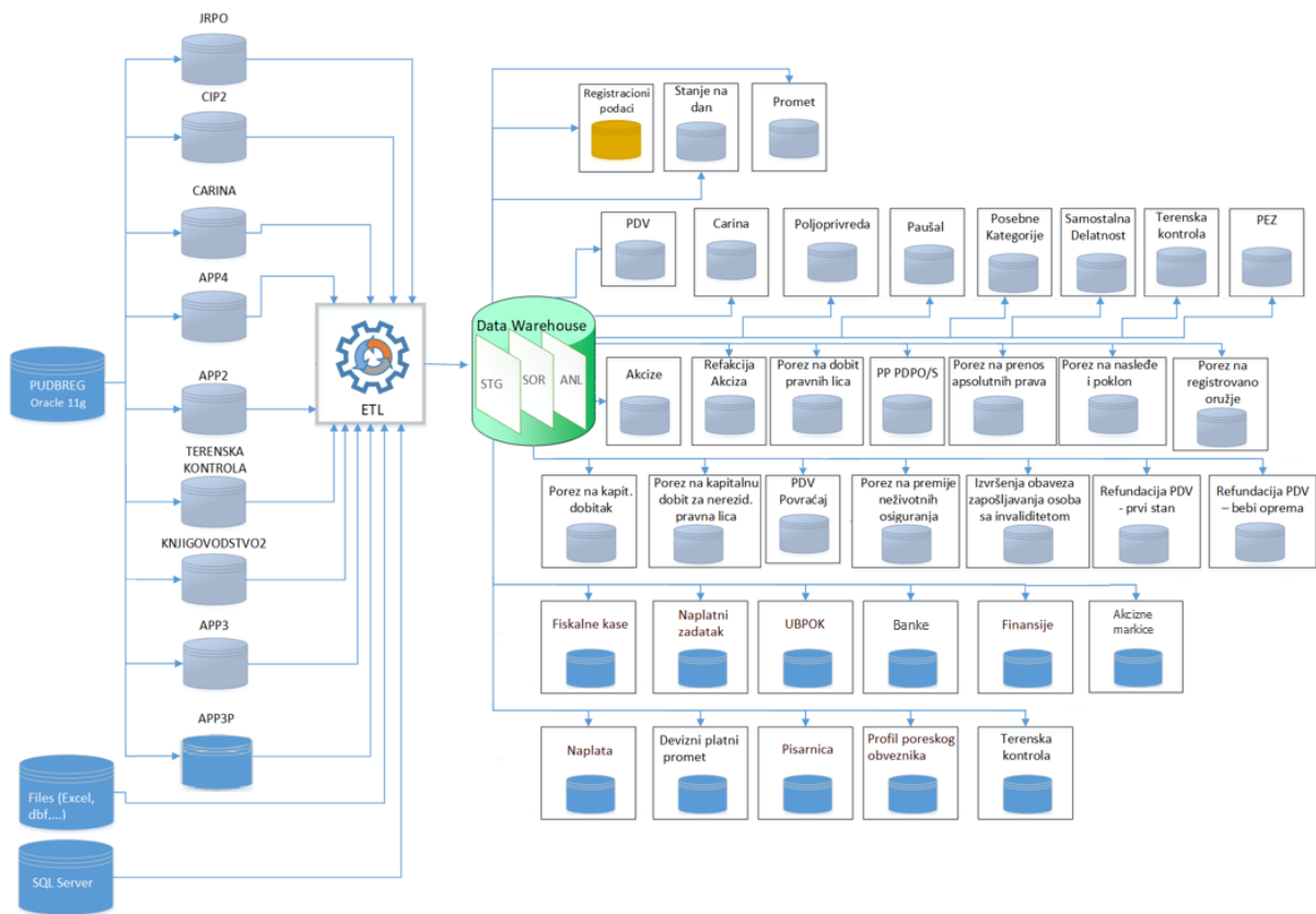
Илустрација 1: Информациона архитектура DWH
