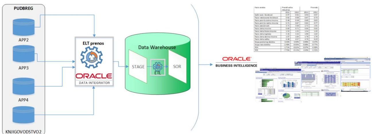
Илустрација 3: Концептуални преглед ETL процеса преноса података
